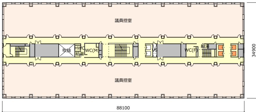
4階平面図
