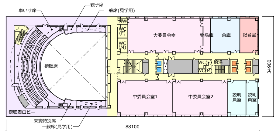
6階平面図
