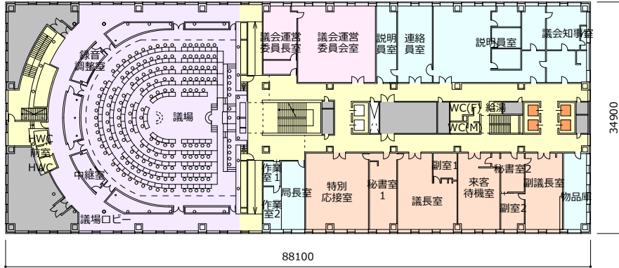
5階平面図
