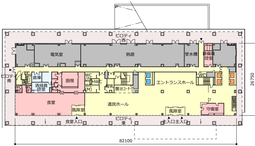
1階平面図
